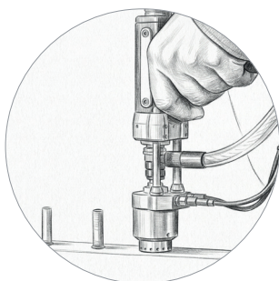
Bolzenschweißen
