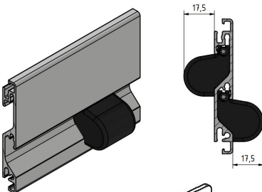
SG-Griff rund (2 Stück)
