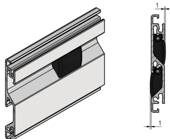
SG-Griff flach (2 Stück)
