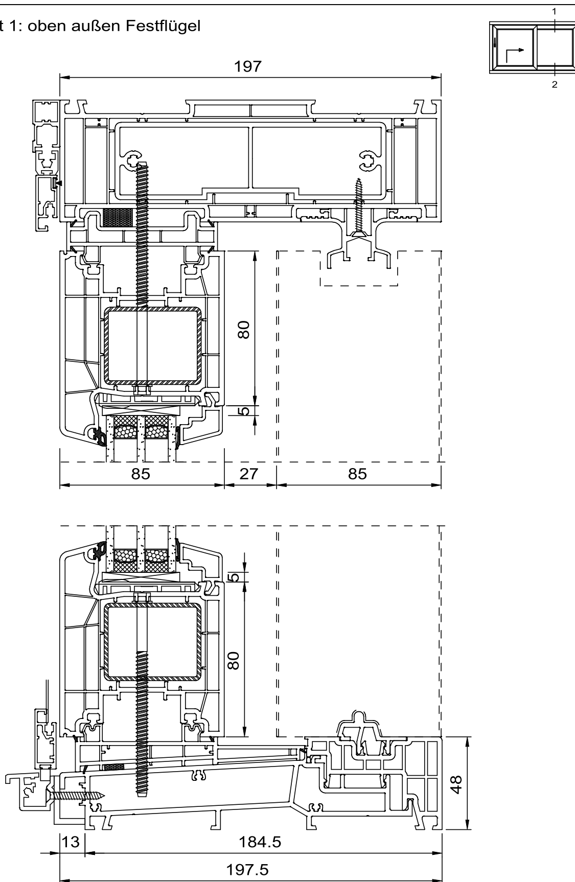
Schnitt 2 : unten außen Festflügel
