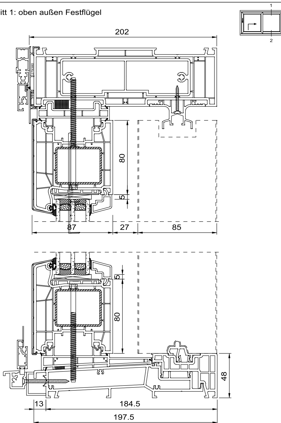
Schnitt 2 : unten außen Festflügel
